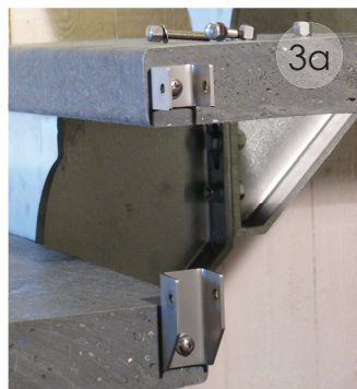
3a Version VF3: Attachez le set de fixation contre l'escalier.
